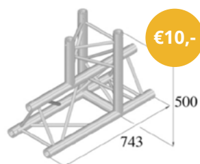
Pro-Truss 33 T-stuk C370 3-weg T-stuk
