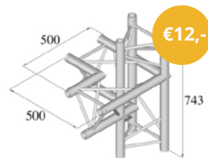
Pro-Truss 33 hoek C440 4-weg hoek
