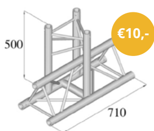
Pro-Truss 33 T-stuk C350 3-weg T-stuk
