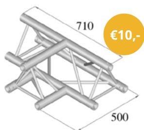
Pro-Truss 33 T-stuk C360 3-weg T-stuk
